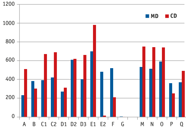
Abbildung 3: Bruchdehnung [%]
