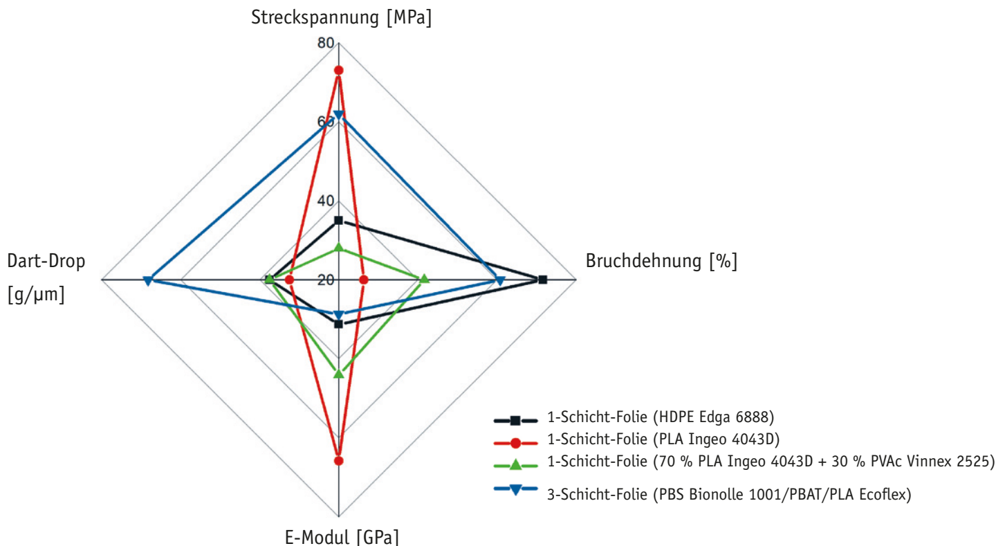
Abbildung 2: Vergleich der Eigenschaften un- und modifizierter Biokunststofffolien
