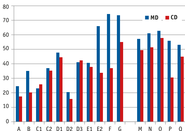
Abbildung 2: Maximale Zugfestigkeit [MPa]
