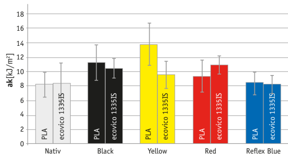
Abbildung 2: Schlagzähigkeitsergebnisse nach 14-tägiger UV-Bestrahlung
