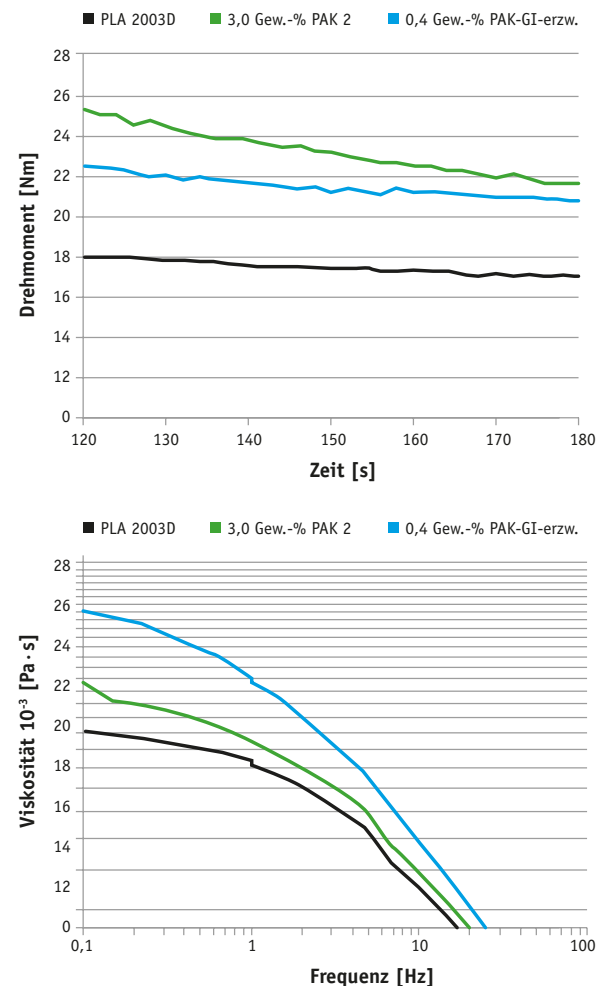
Abbildung 1: Rheologische Kurven von chemisch und physikalisch modifiziertem PLA
