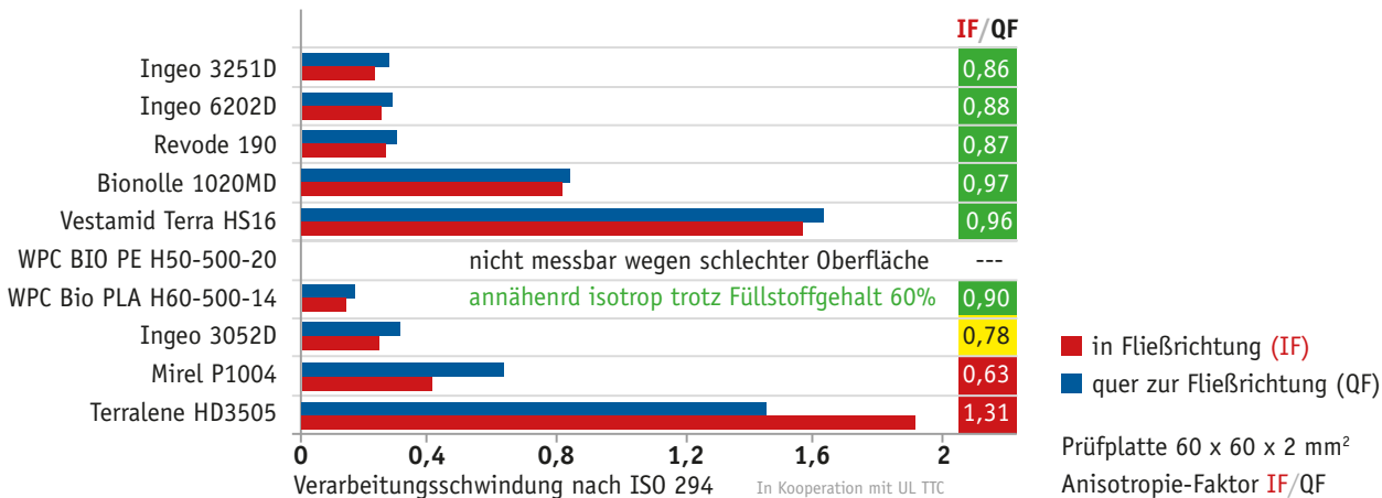
Abbildung 2: Schwindung und Verzug von Biokunststoffen
