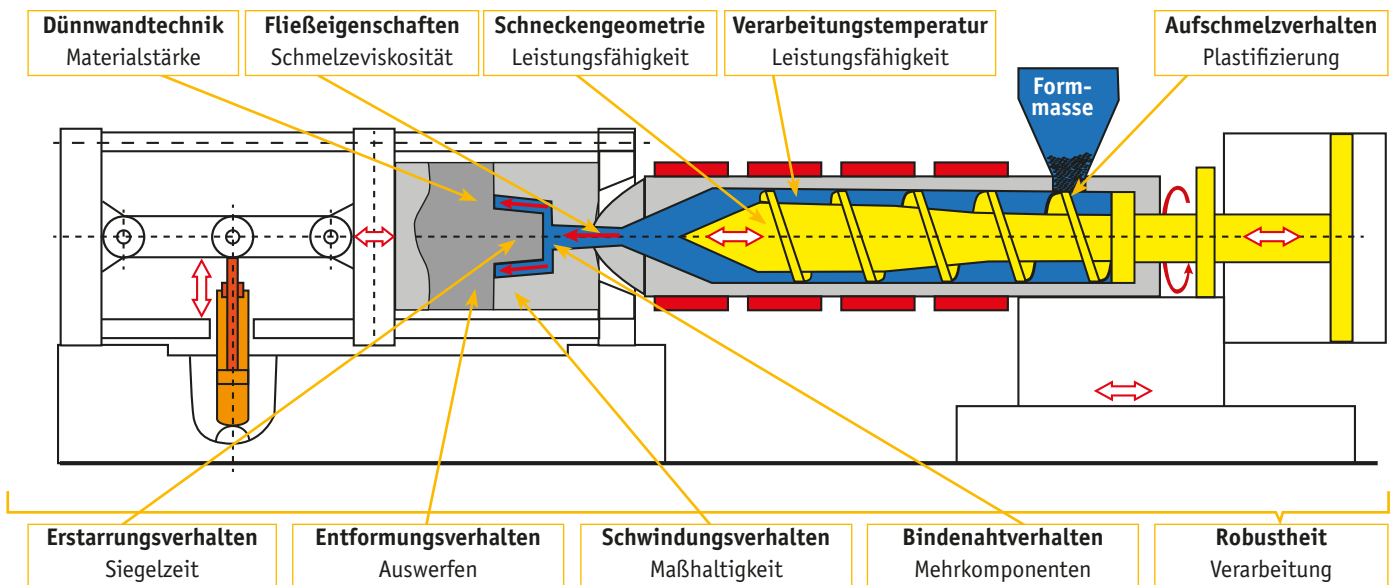
Abbildung 1: Faktoren mit Auswirkungen auf den Spritzgießprozess
