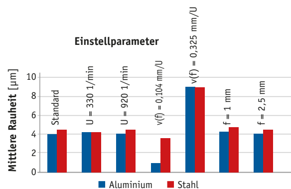
Abbildung 2: Mittlere Rauheit von Ingeo 3251D abhängig von den Einstellparametern
