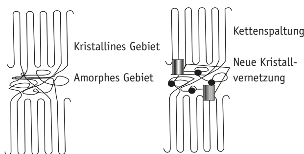
Abbildung 1: Wirkung von Strahlenvernetzung auf die Morphologie eines nicht bestrahlten und eines bestrahlten teilkristallinen Polymers
