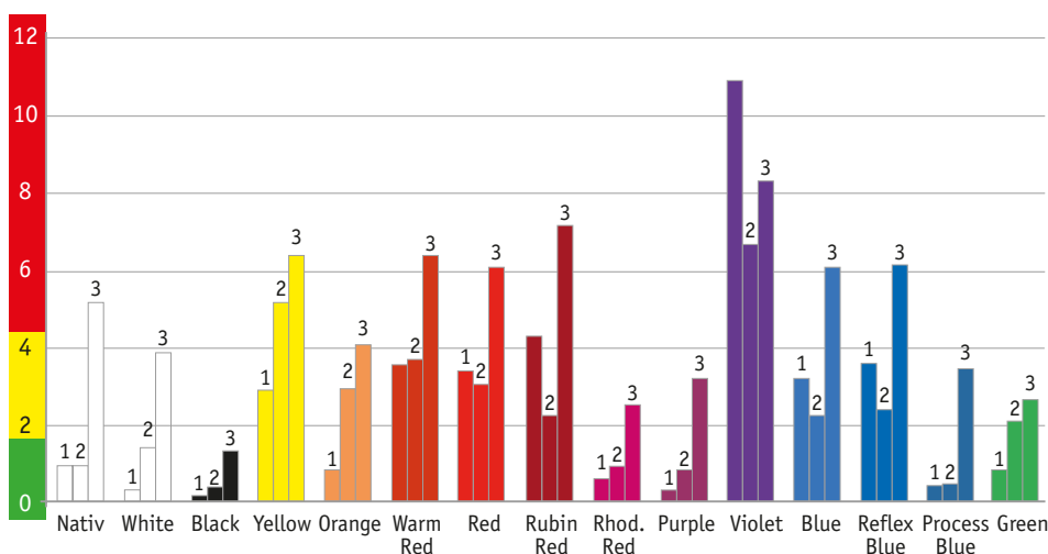
Abbildung 1: Farbabstand nach 14-tägiger UV-Bestrahlung
