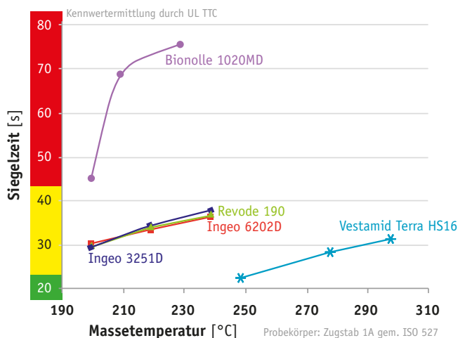
Abbildung 4: Siegelzeiten von Biokunststoffen
