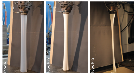
Abbildung 1: Vorformlingsbildung im Extrusionsversuch
