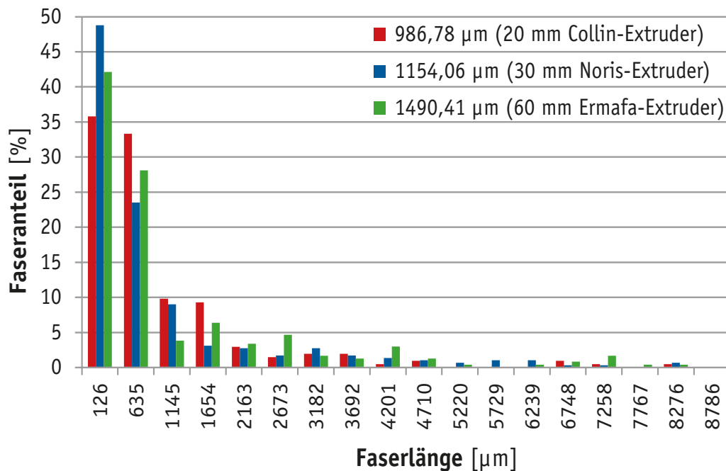
Abbildung 2: Faserlängenverteilung und durchschnittliche Faserlänge in Abhängigkeit des Schneckendurchmessers
