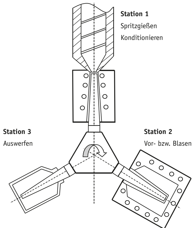
Abbildung 1: Spritzblasformen
