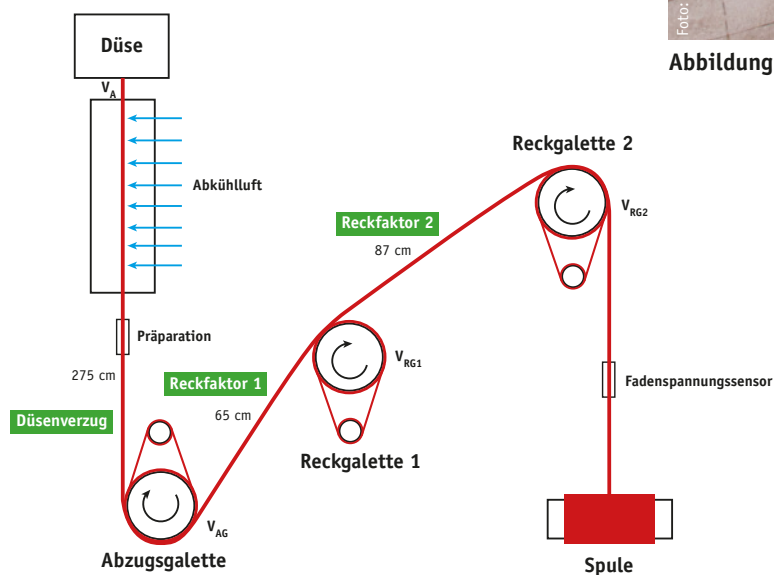
Abbildung 1: Filamentgarnverlauf des Verspinnprozesses
