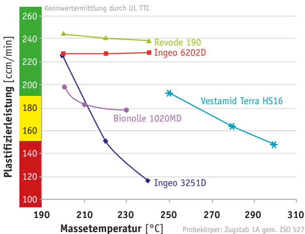
Abbildung 3: Plastifizierleistung von Biokunststoffen
