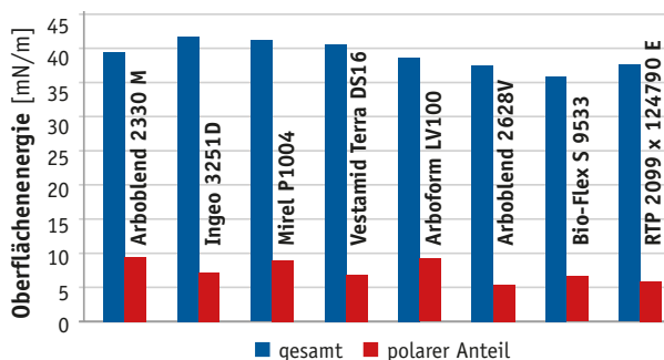
Abbildung 1: Oberflächenenergie
