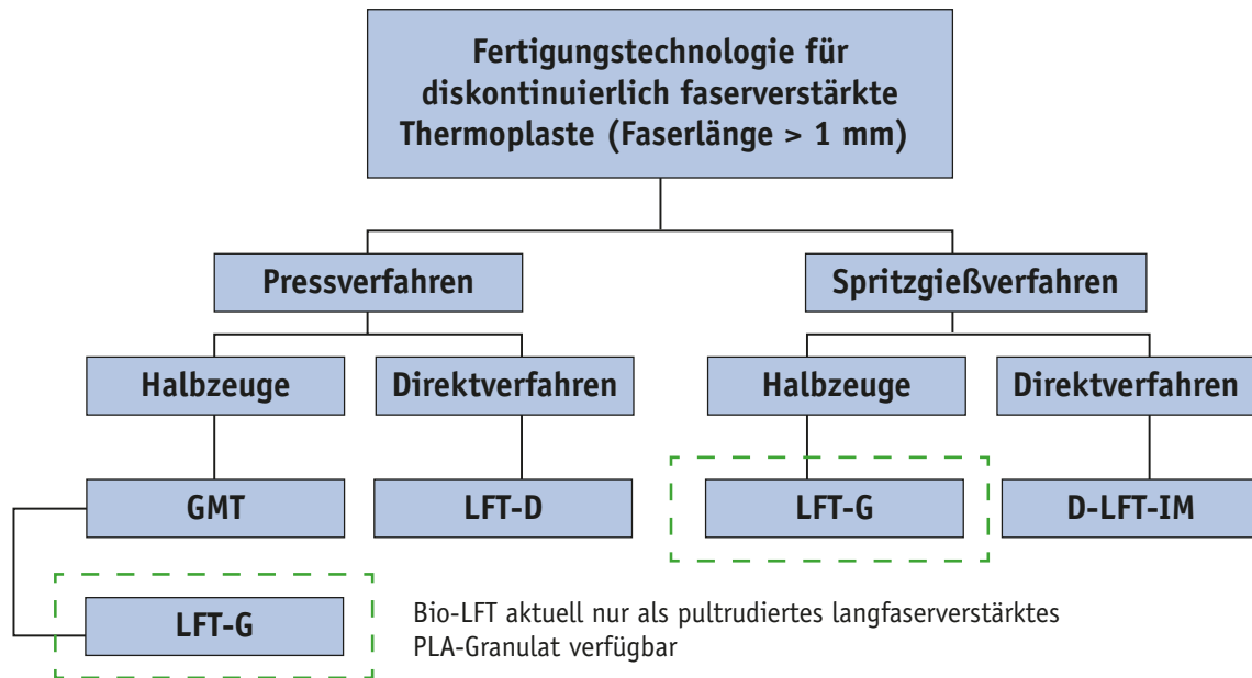
Abbildung 1: Gliederung der Fertigungstechnologien für langfaserverstärkte Thermoplaste
