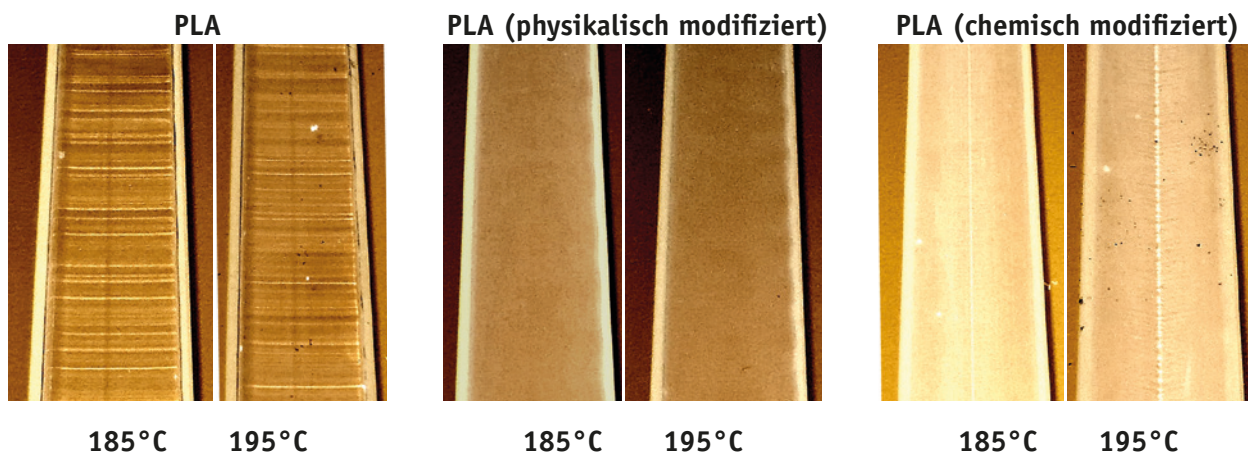
Abbildung 2: Extrudierte Profile von unmodifiziertem und modifiziertem PLA
