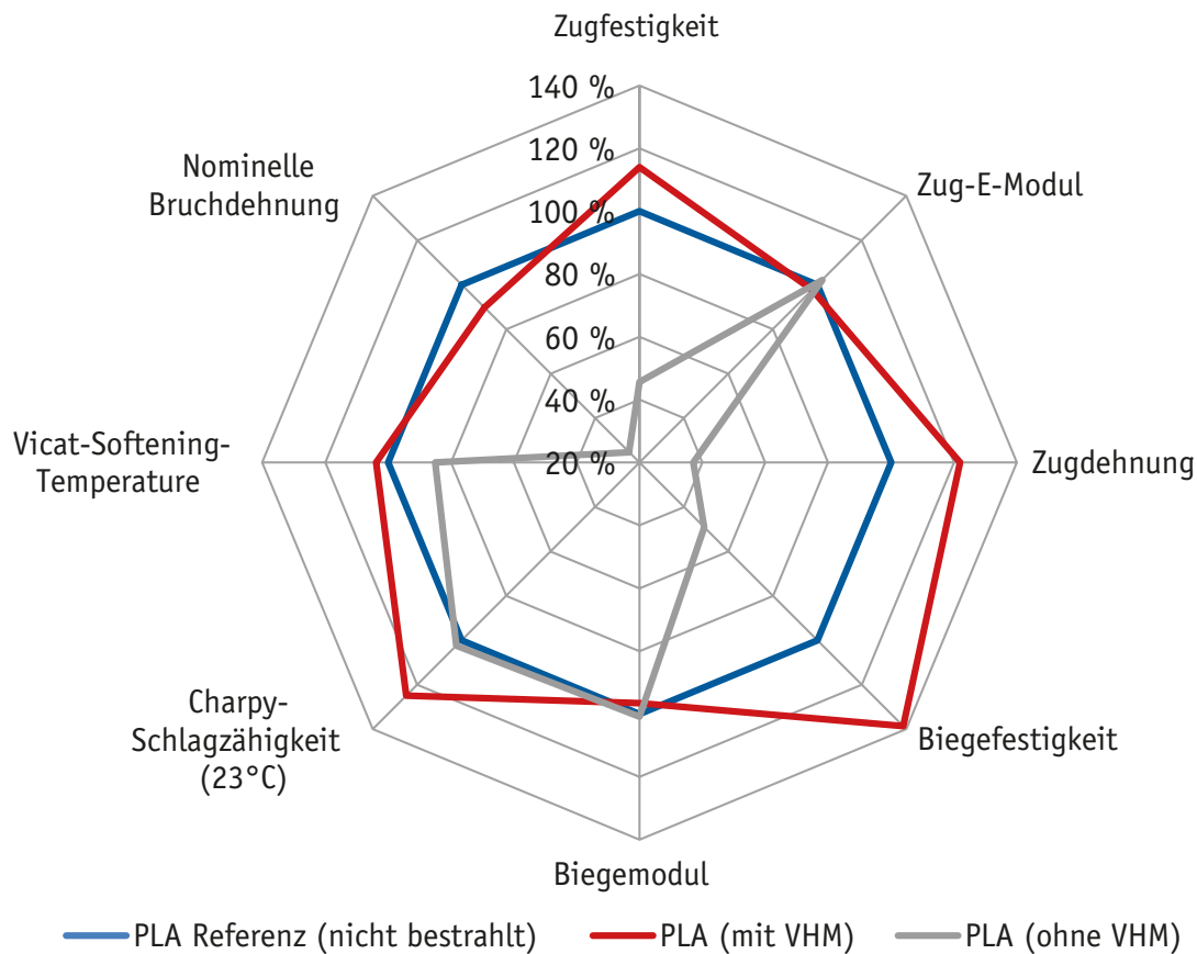
Abbildung 2: Einfluss durch Bestrahlung auf die Eigenschaften von PLA
