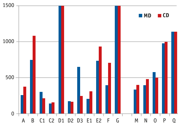
Abbildung 1: E-Modul [MPa]
